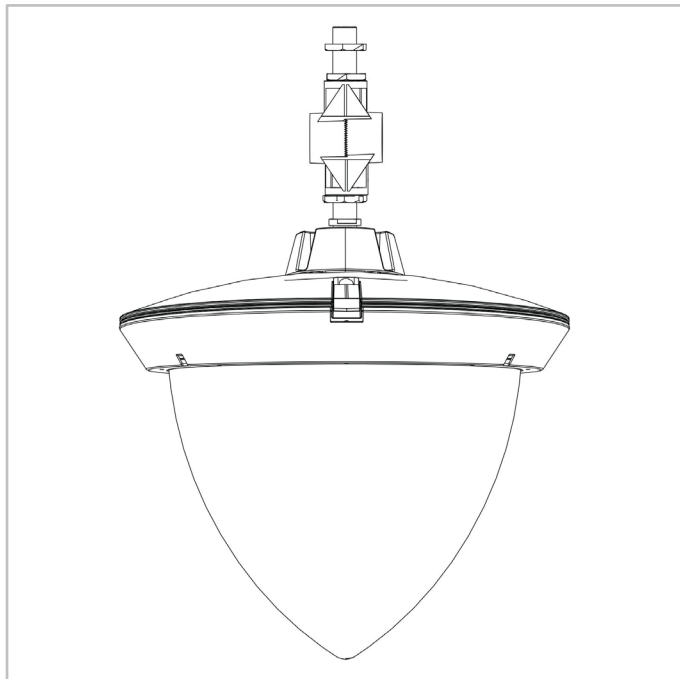
FLEXIA QUERCUS | Regulowany zwieszany 1" żeński
