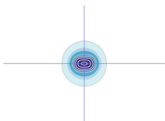
7051 Rozsył światłości 17°
