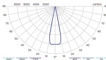
7050 Rozsył światłości 25°
