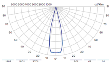
7049 Rozsył światłości 30°
